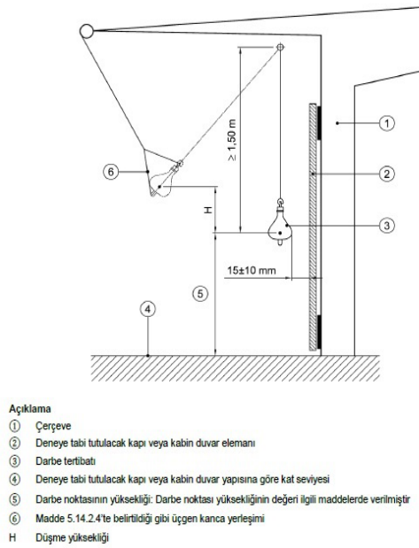
Resim 3: Yumuşak darbe deney cihazı
