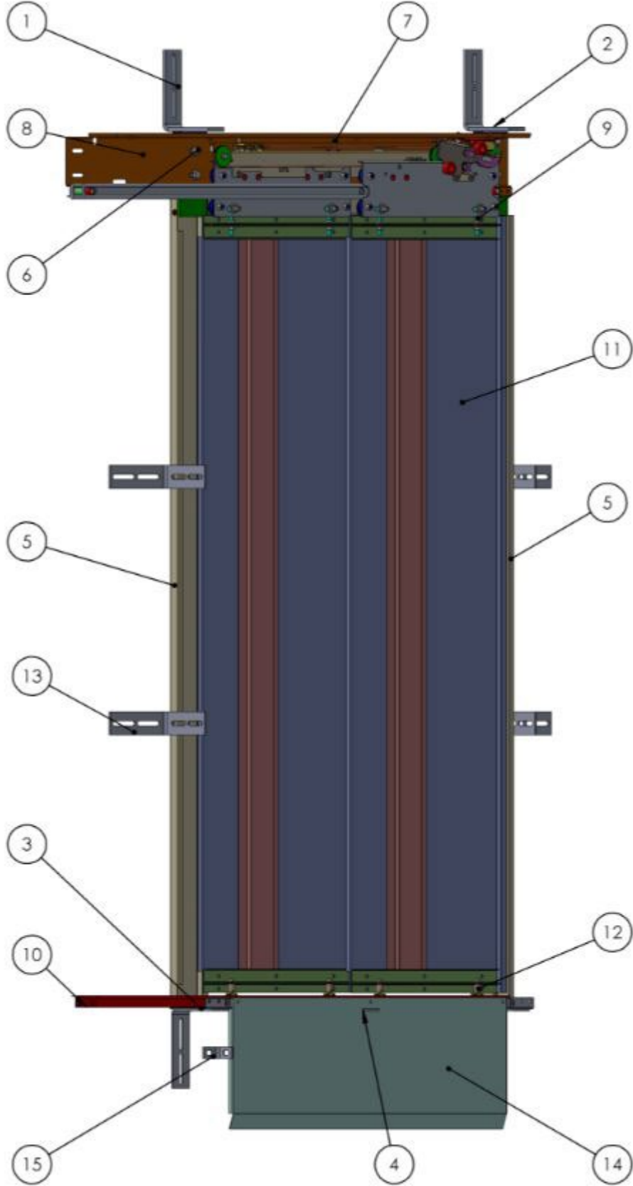
Resim 1: Teleskopik Durak Kapı Montaj Detay
