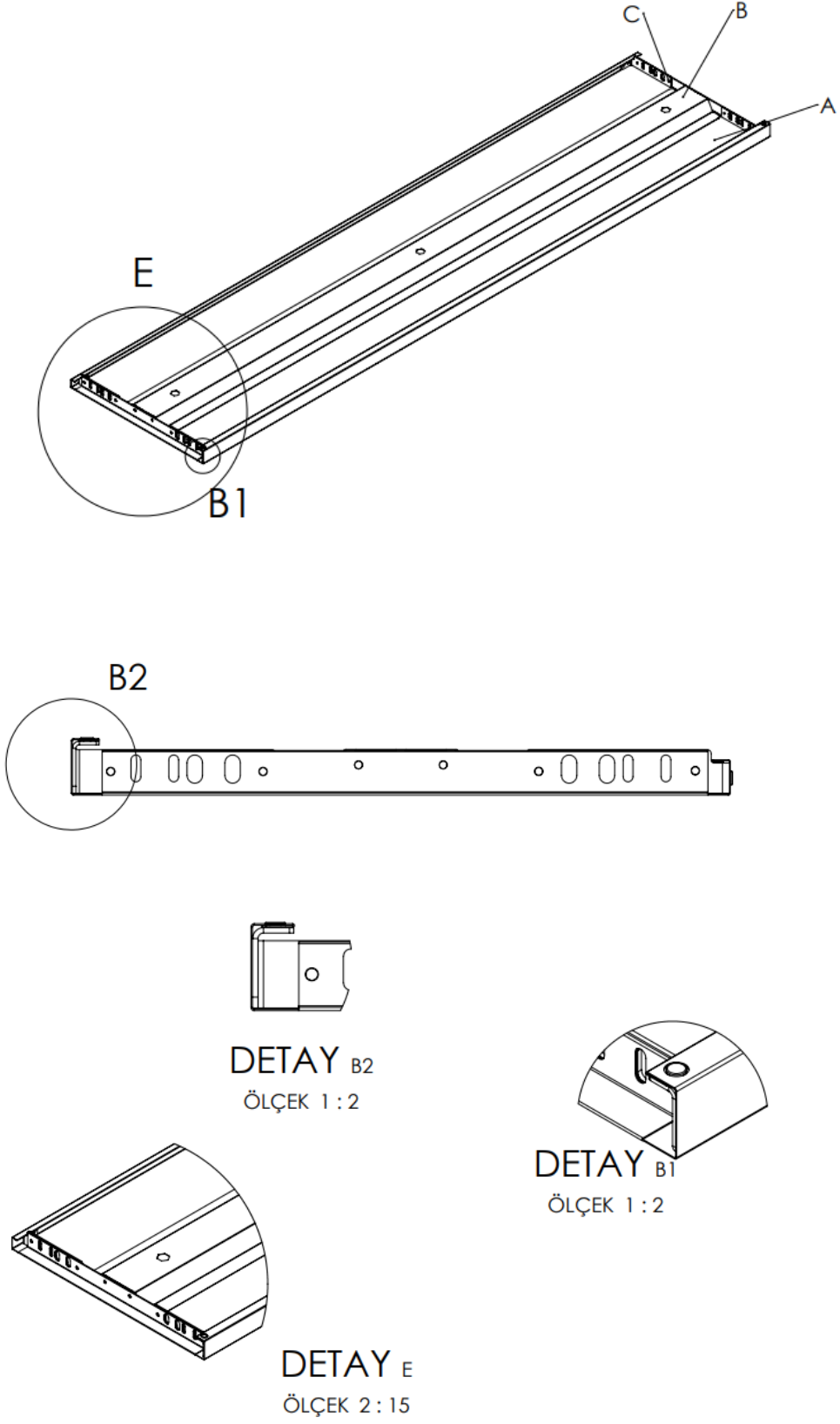
Resim 3: Durak Kapısı Paneli Detay
